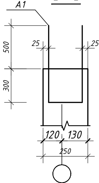
2 - 2
