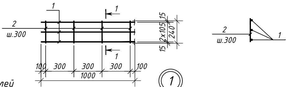
Арматурная сетка СГ1 (разработана на 1 пог.м. длины)
