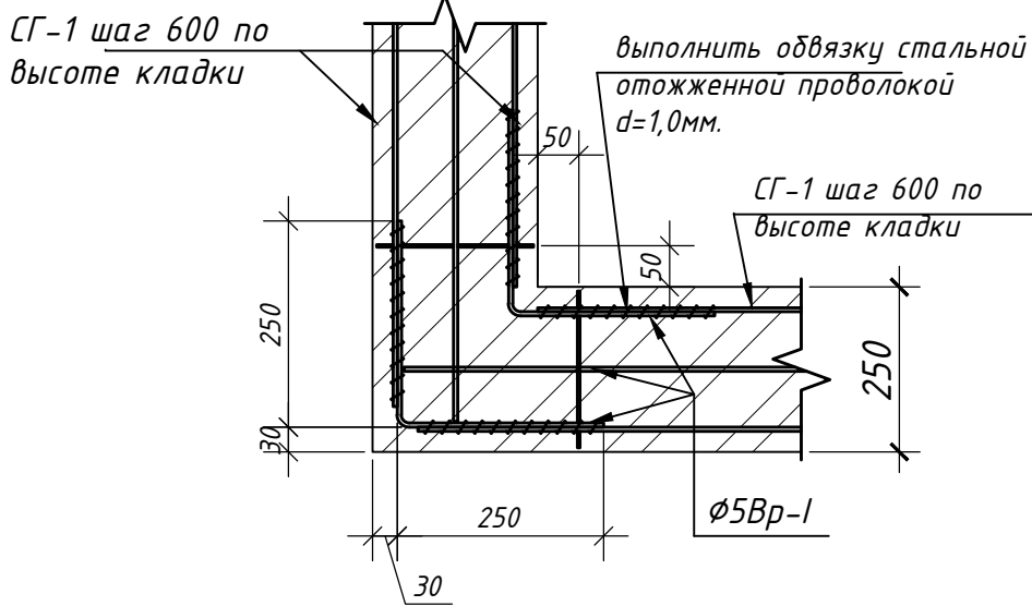
А л.АС-2
