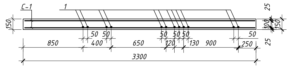
Монолитная Балка Б-1
