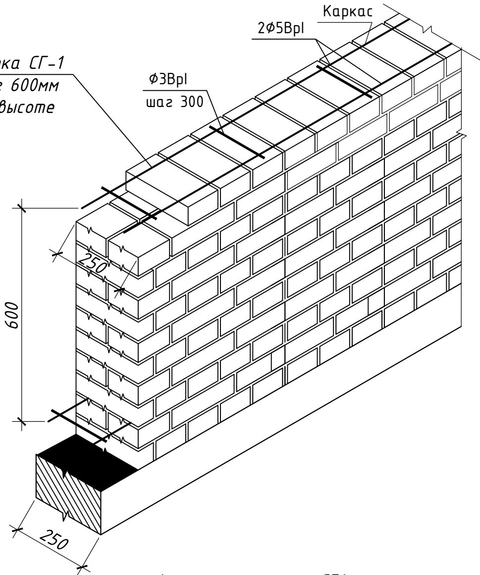
Арматурная сетка СГ1 (разработана на 1 пог.м. длины)
