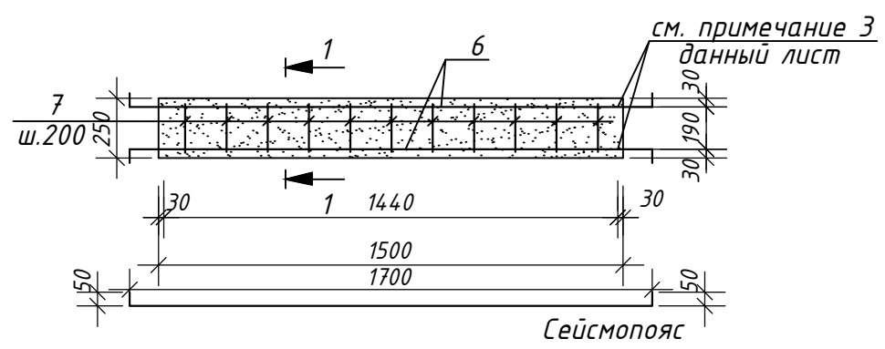
Монолитная Балка Б-1
