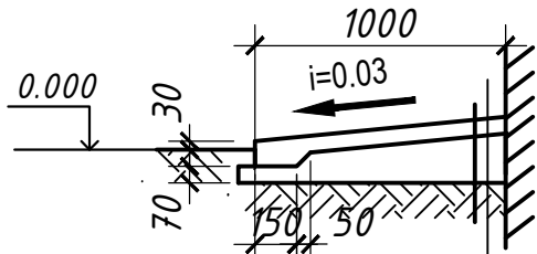
Деталь отмостки
